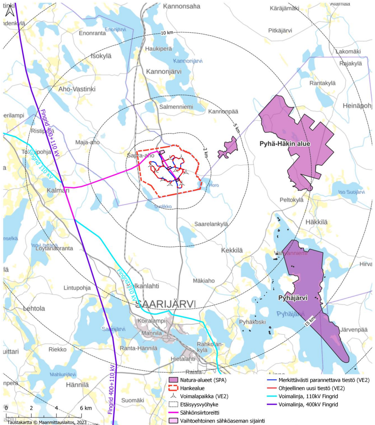
Kuva 3. Karstulan Tukkimäen tuulivoimapuiston vaihtoehto 2 (VE2): toteutetaan 9 voimalan hanke. Kuvassa esitetään suunnittelualue, voimalapaikat, niille johtava tiestö, sähkönsiirtolinjat ja lähimmät Natura-alueet (Pyhä-Häkki ja Pyhäjärvi).
