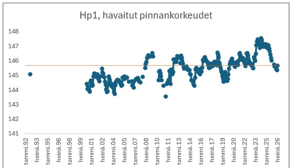
Kuva 2. Mittauspisteen Hp1 pohjaveden pinnantasoo ajanjaksolla syyskuu 1992 – elokuu 2026. Pohjaveden pinnankorkeuden yksikkö on metri (m) korkeusjärjestelmässä N2000. Oranssi viiva on pohjaveden pinnantasoo tällä hetkellä.
